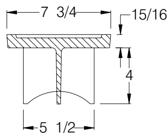
LID 4002
