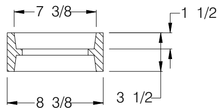
COLLAR 4004
