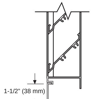
Flange Frame
