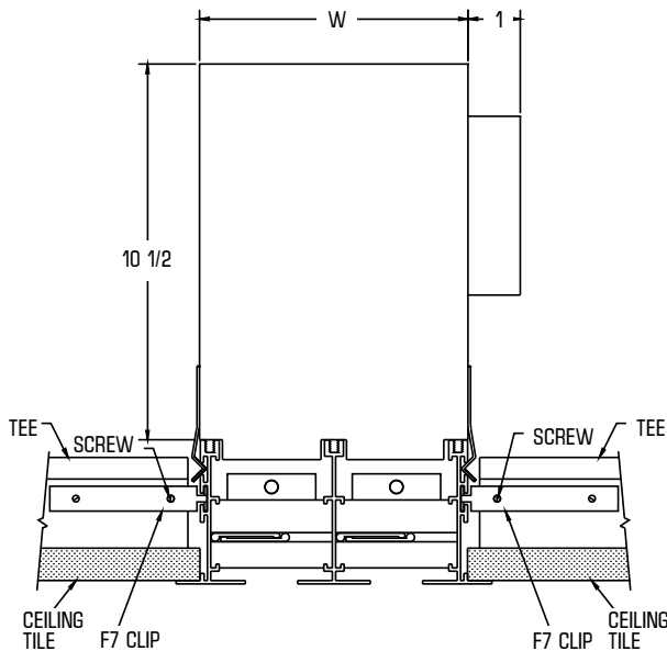
2 SLOT
