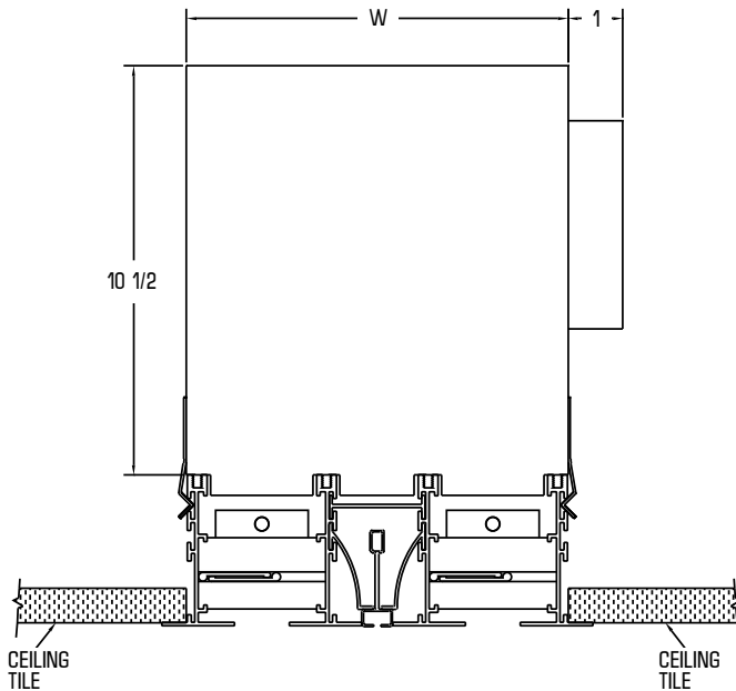
2T SLOT
