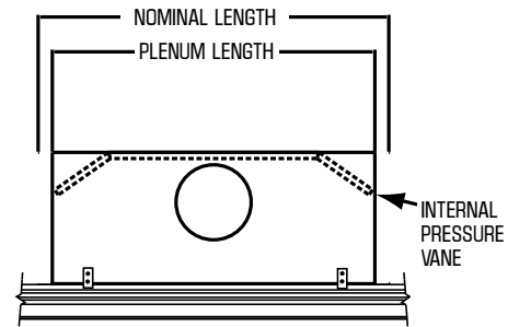
PLENUM SIDE
