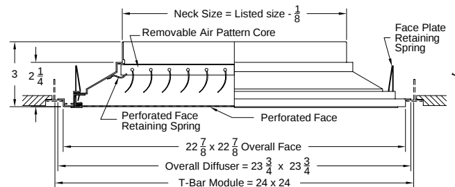
Model: 7000-8 ( Tegalur T-Bar )
