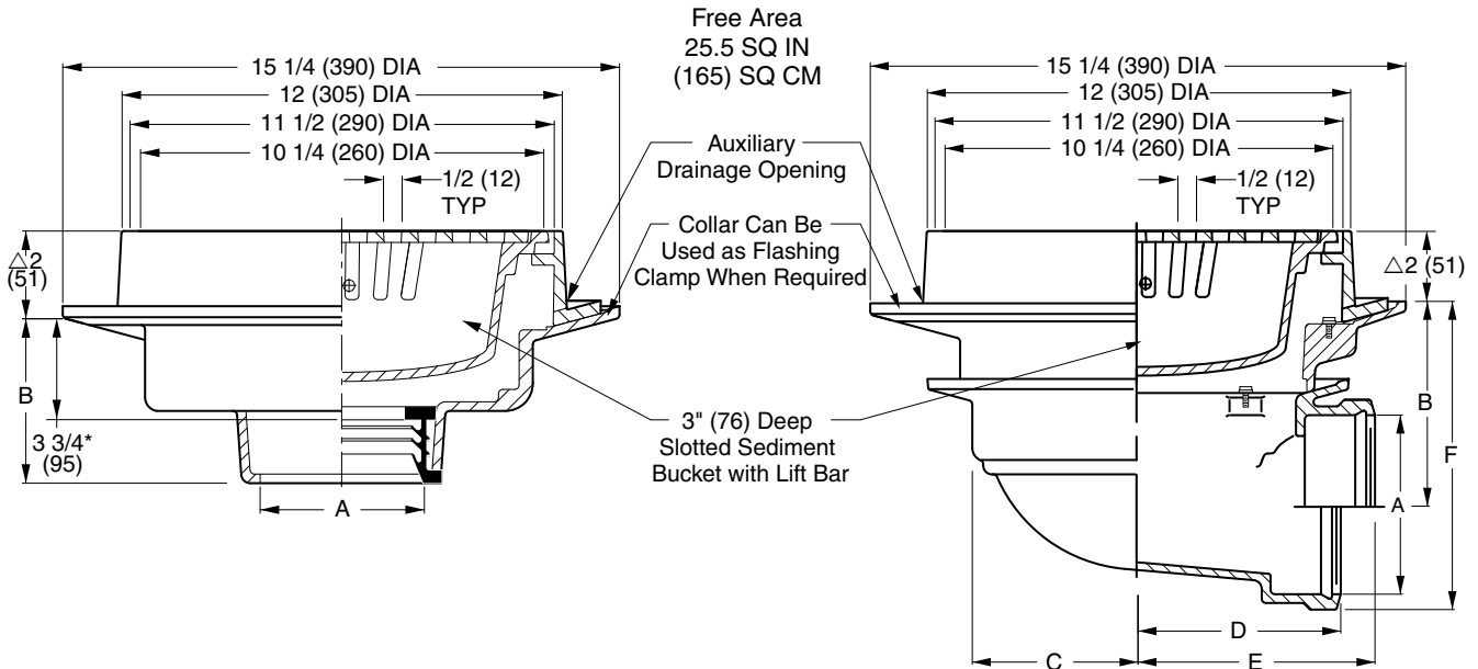
Fig. 2230C.....CAULK OUTLET Fig. 2230Y.....NO-HUB OUTLET
