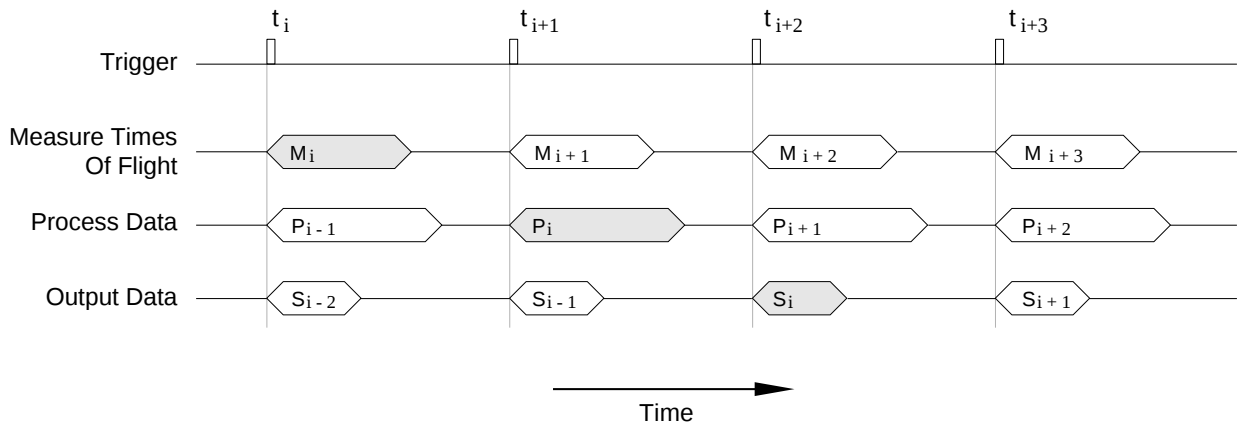
FIGURE 9-1. CSAT3 Pipeline Delay
