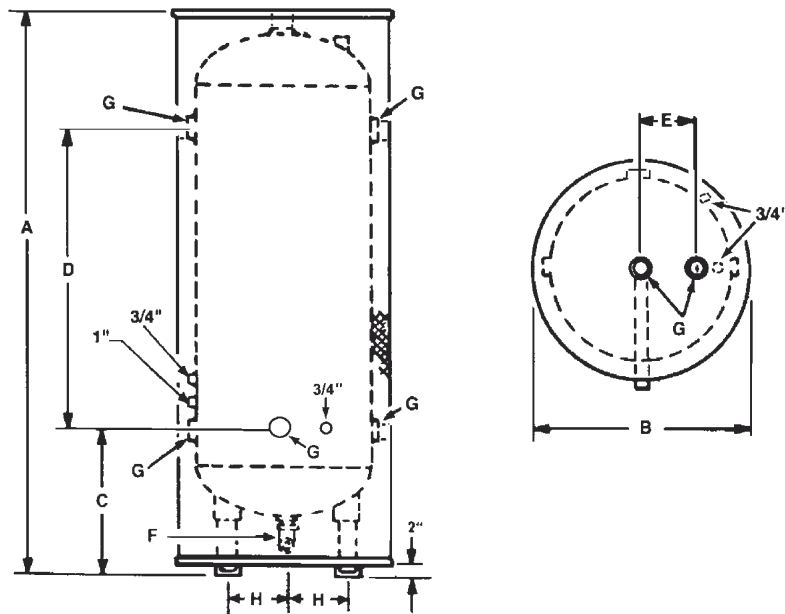
TJV-140 THRU TJV-1000
