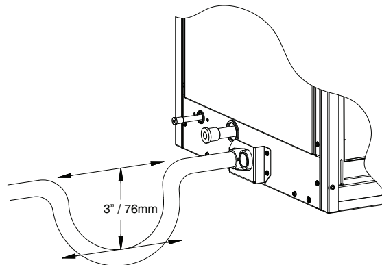
Fig. 8 - Condensate Trap
